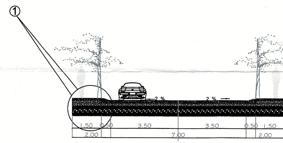
SECCION CALLE SECUNDARIA
